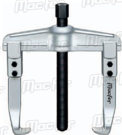
SACA ROLAMENTOS 2 PERNAS MOVÍVEIS TD0804
