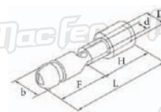
TERMINAL CABO ELÉCTRICO ISOLADO BALA MACHO TBMi
