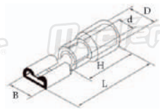
TERMINAL CABO ELÉCTRICO ISOLADO PLANO FÊMEA TPFi
